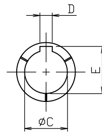
INPUT SHAFT
