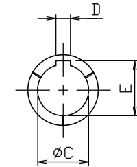
INPUT SHAFT
